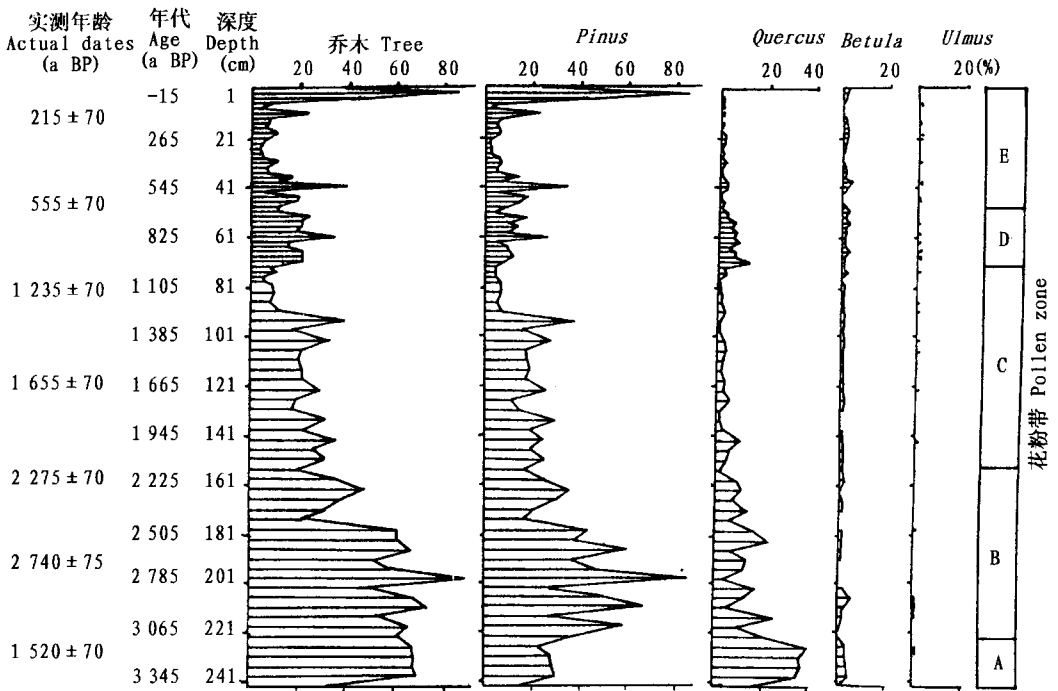
图3 麦里泥炭剖面化石花粉百分比 Fig.3 Pollen percentages for Maili section
