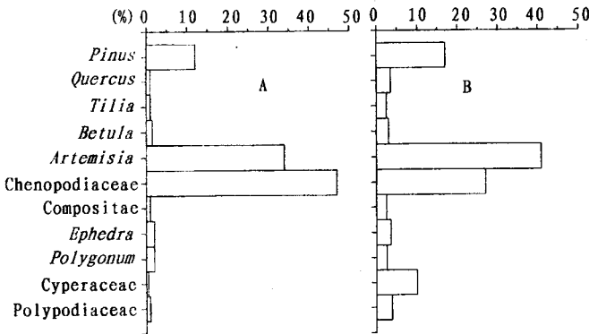
图 2 麦里地区土壤(A)和沼泽(B)表层主要种类花粉百分比 Fig. 2 Modern pollen percentages of soil (A) and bog (B) for Maili region
